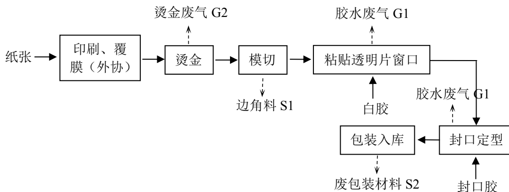
图 2-3 卡纸盒生产工艺流程与产污图
