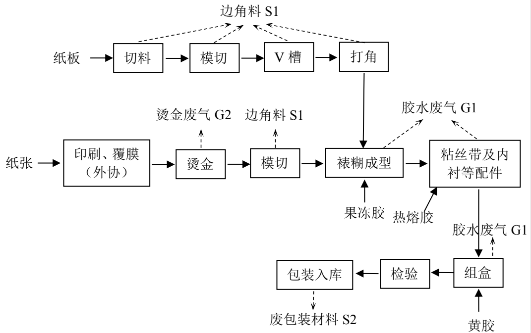
图 2-2 礼盒生产工艺流程与产污图
