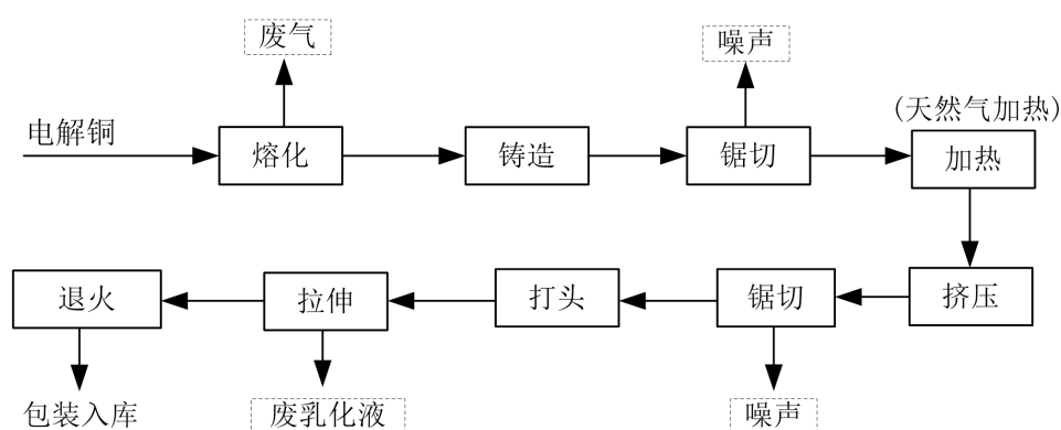
图 4.1-1 紫铜管生产工艺流程图
