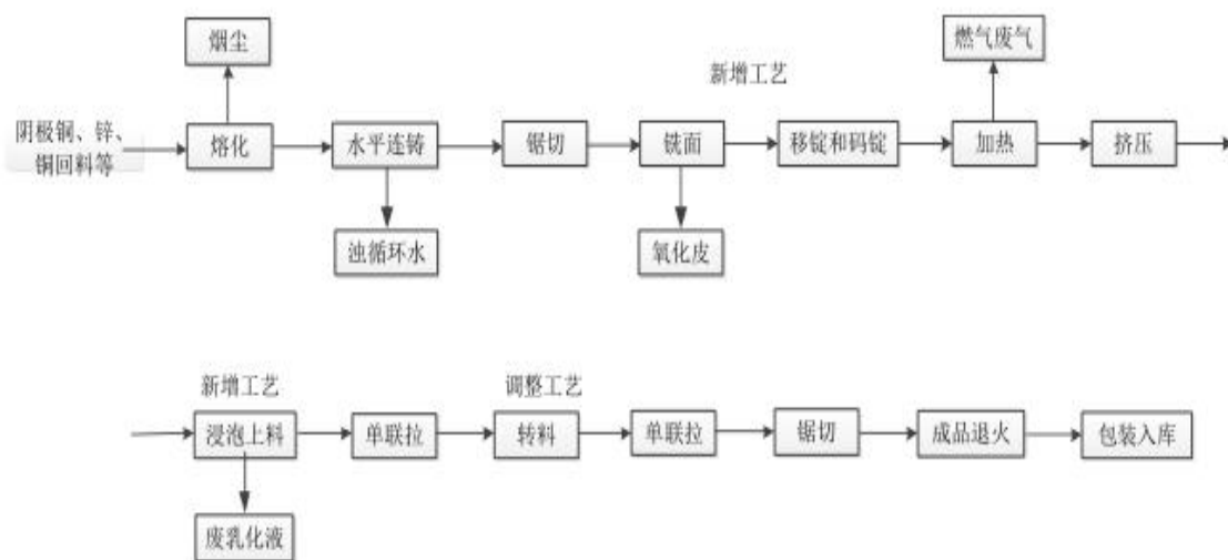
图 2.1-5 铜合金冷凝管生产工艺流程图
