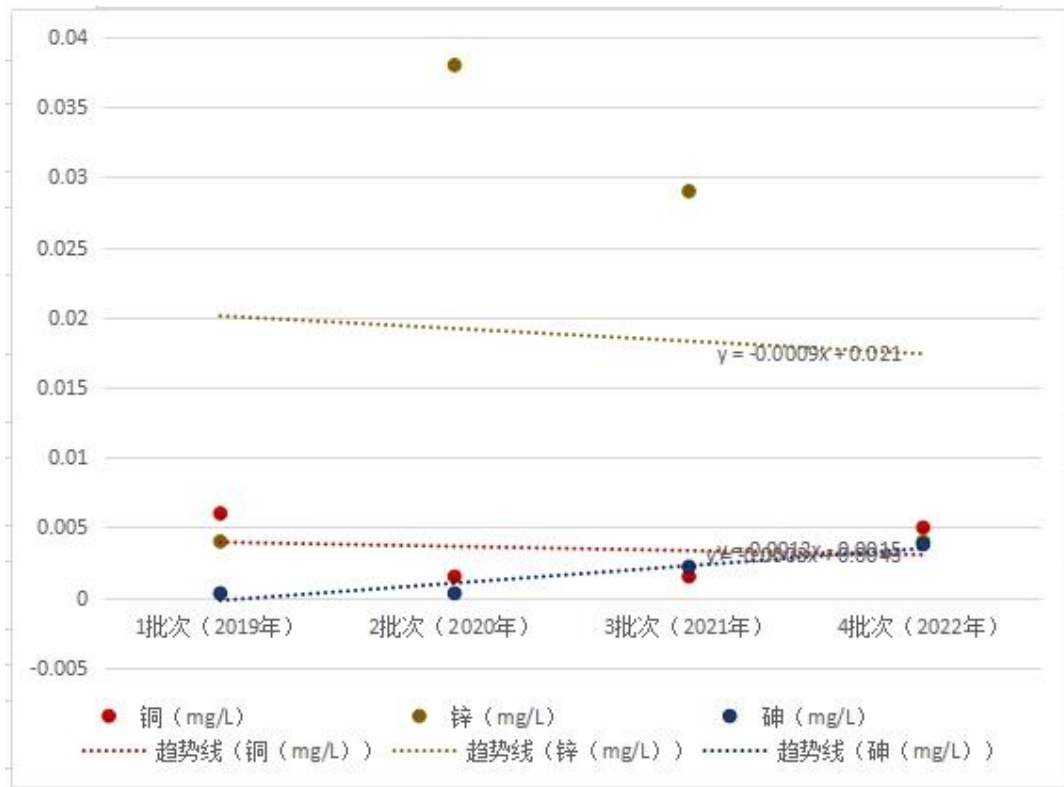
图 8.2-1 监测井 BS1 污染物趋势图
