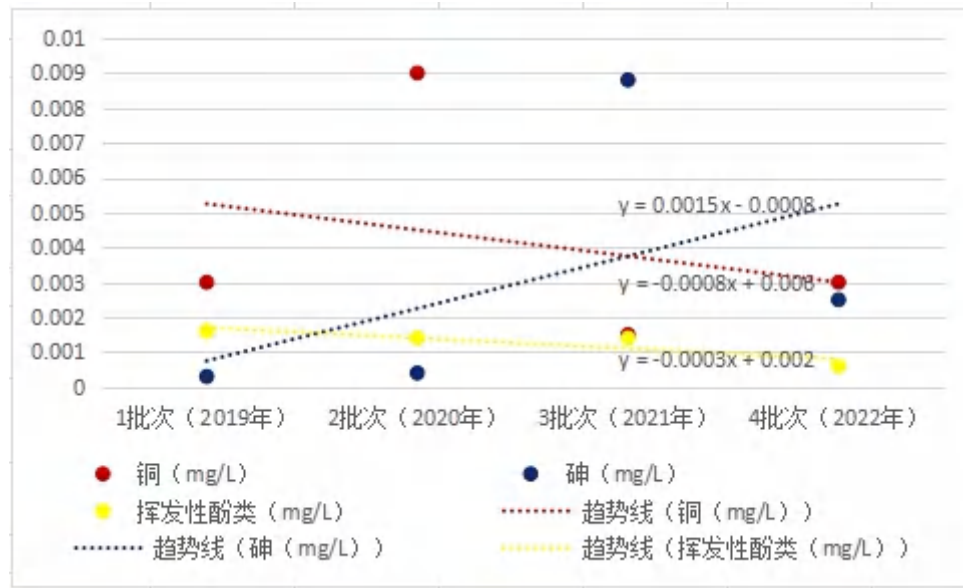
图 8.2-3 监测井 FS1 污染物趋势图
