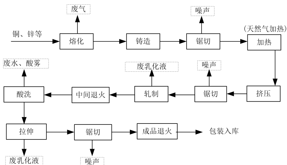
图 4.1-2 黄铜管生产工艺流程图
