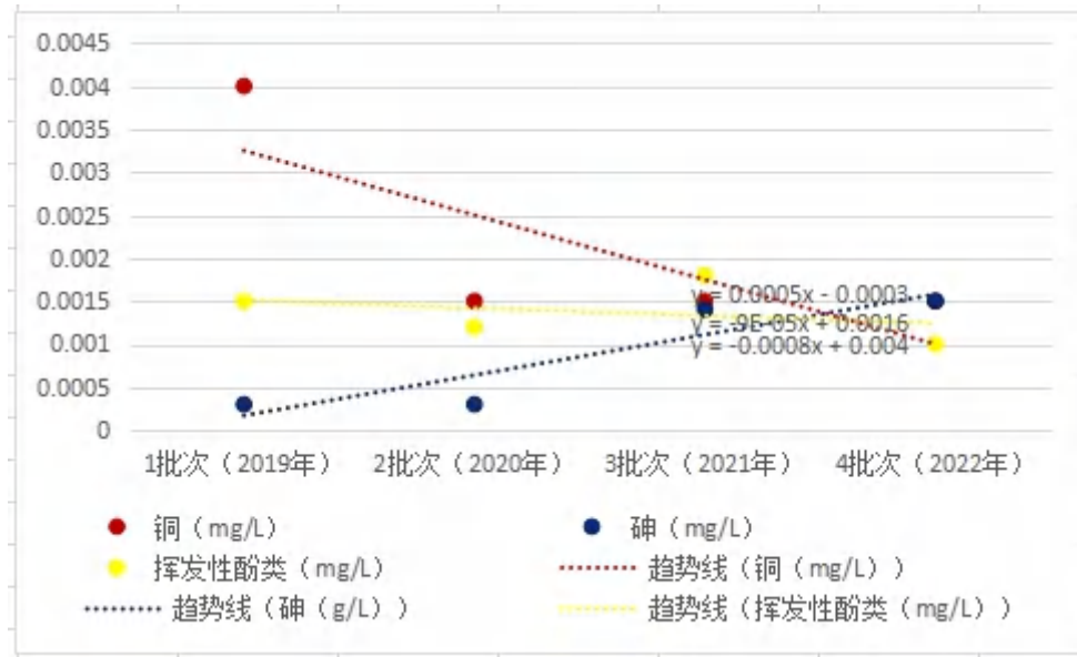
图 8.2-2 监测井 ES1 污染物趋势图
