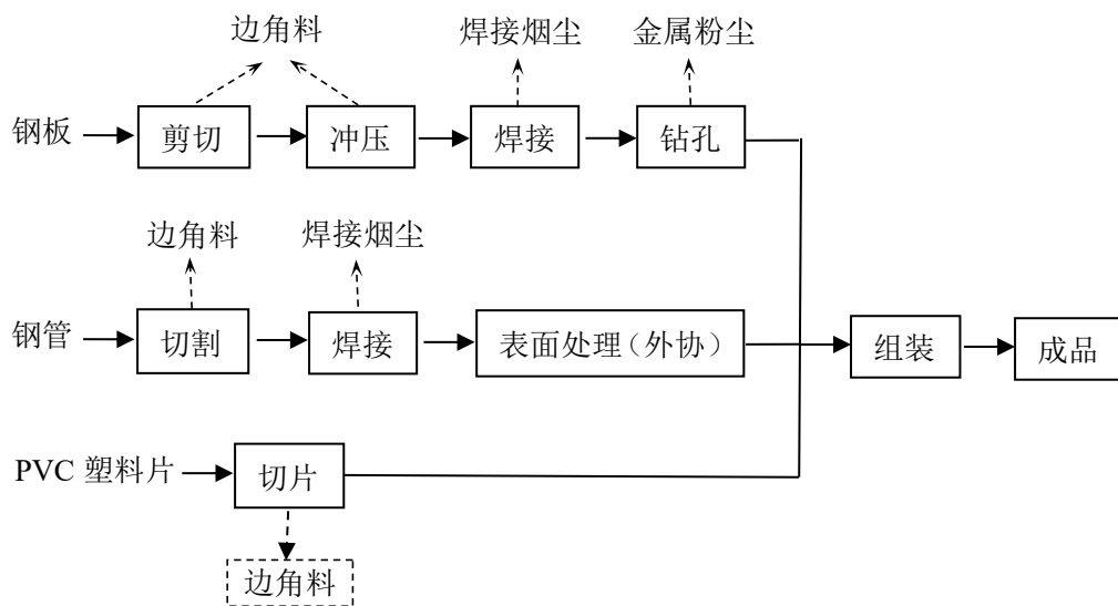
图 2-6 生产工艺流程与产污图
