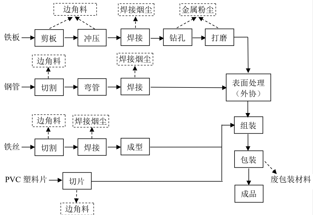
图 2-3 铁质类广告产品生产工艺流程与产污图
