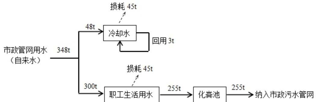
图2-1 全厂水平衡图
