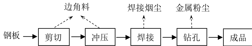
图 2-5 生产工艺流程与产污图
