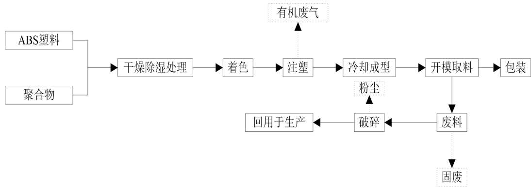
图 2-1 企业注塑生产工艺流程图
