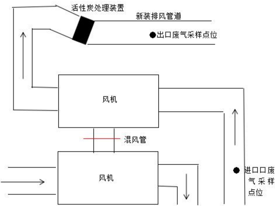
图 4-1 采样检测口位置分布图
